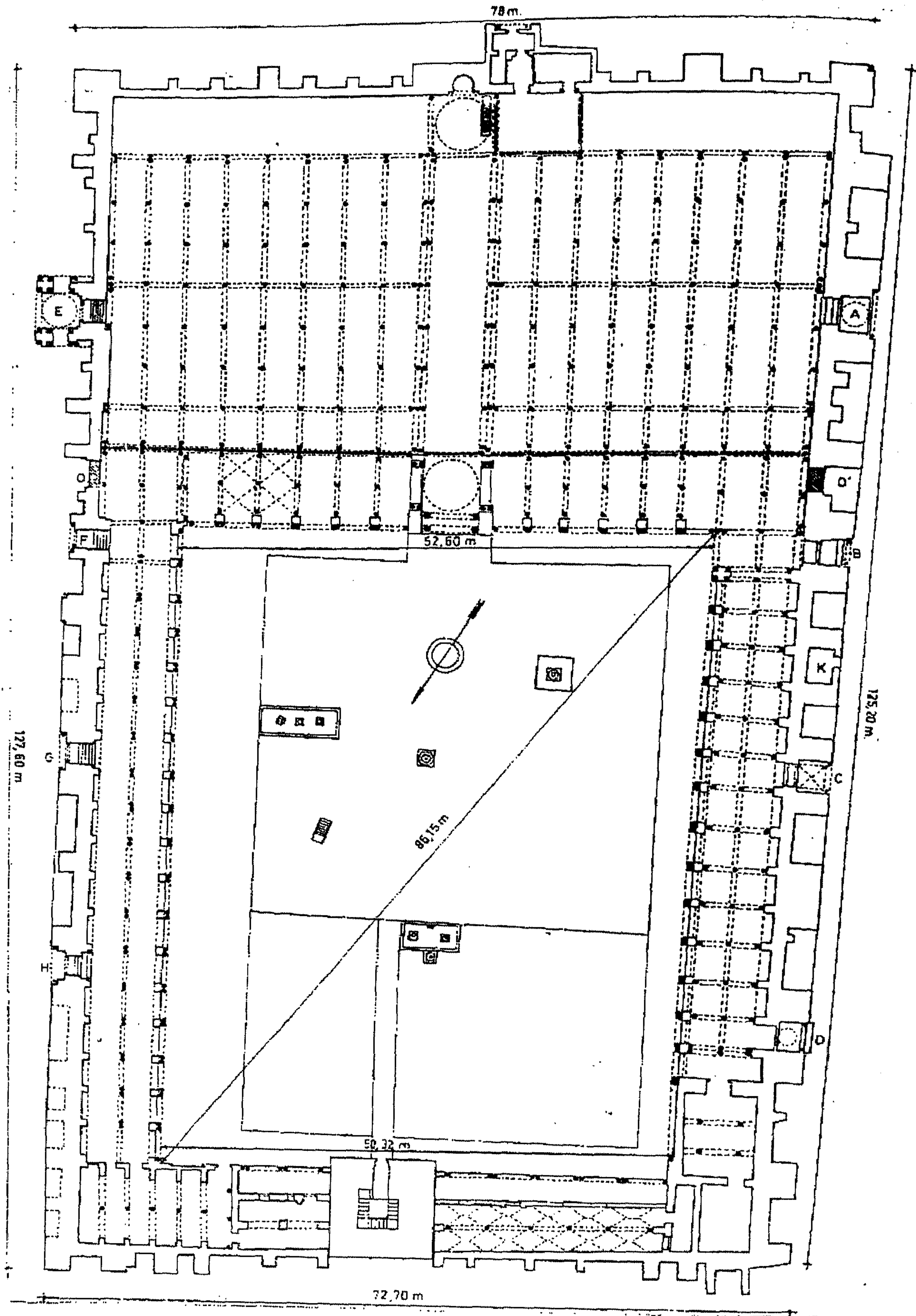
(شكل رقم ١٢) رسم تخطيطي لجامع القيروان بشكله الحالي عن جولفان
